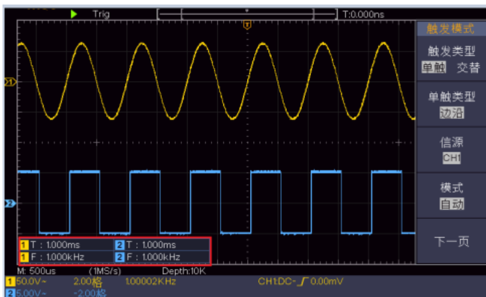
圖 4-12：自動測量
